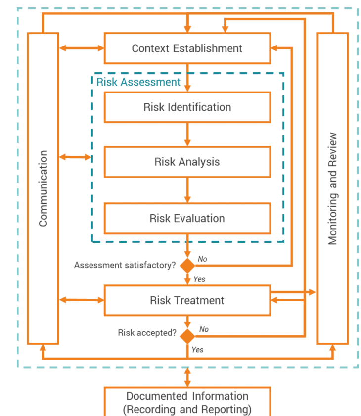
ISO 27005
